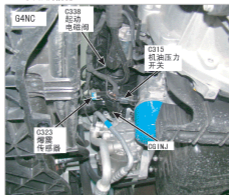
138. 发动机前部
