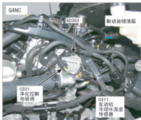
137. 发动机左侧
