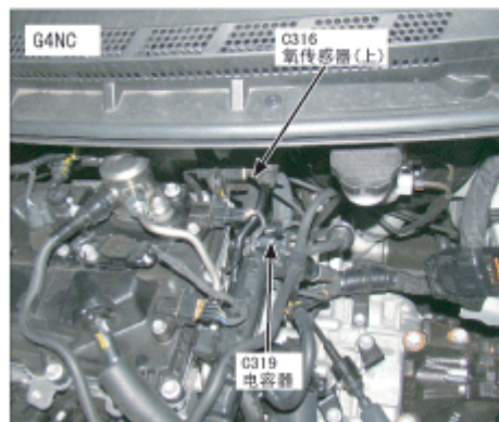
136. 发动机左侧
